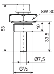
Tauchhülse G \frac{1}{2} x 33
