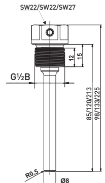
Tauchhülse G \frac{1}{2} B x 85/120/210
