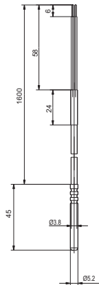
Tauchhülsenfühler THF-45
