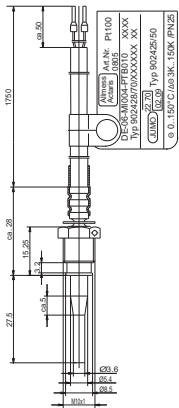
Direkteinbaufühler TDF-27
