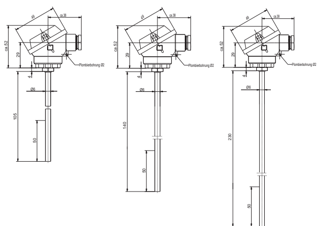
Kopffühler THF-105/140/230
