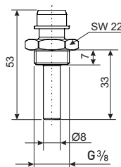
Tauchhülse G \frac{3}{8} x 33
