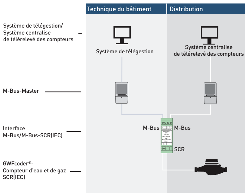
Système de télégestion
